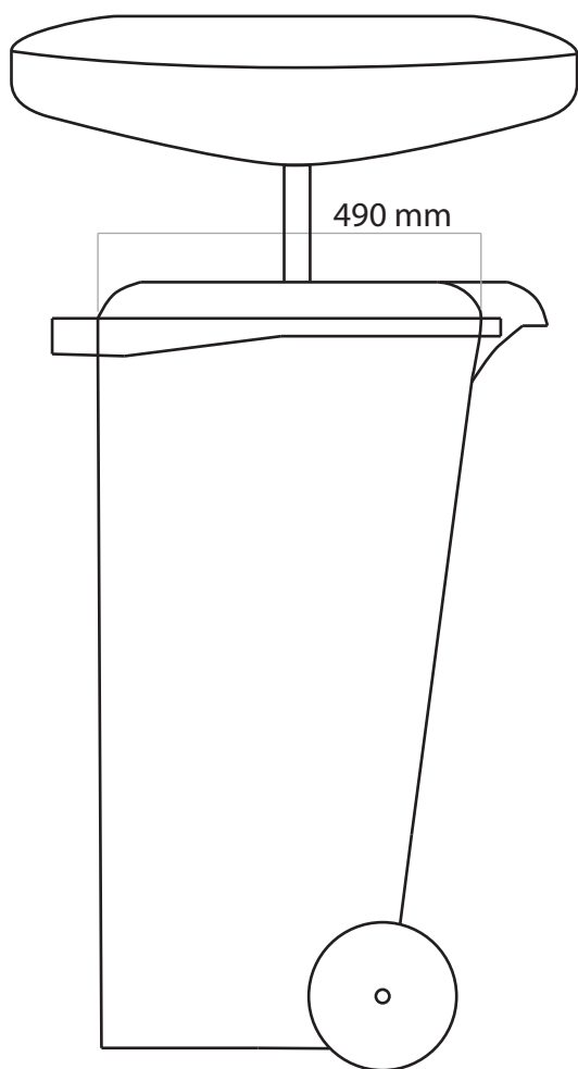
Vista Lateral
